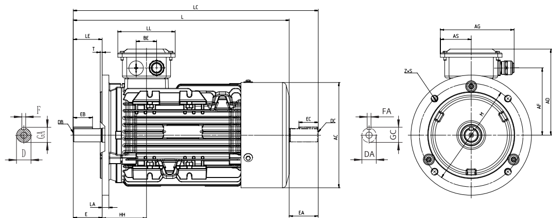
IM B5 以及 IM V1 安装结构型式 Type of construction IMB5 and IMV1
